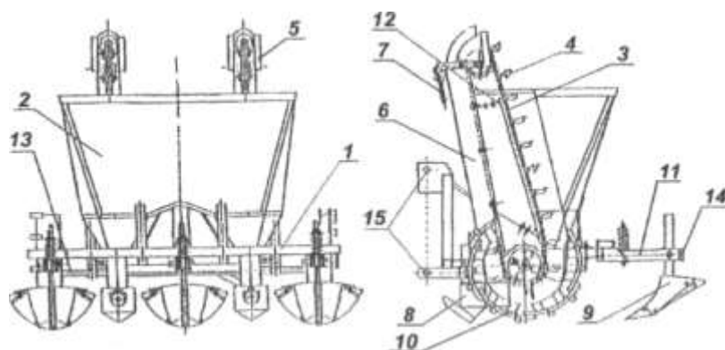
Рисунок 1. Основные узлы конвейерной автоматической сажалки:
